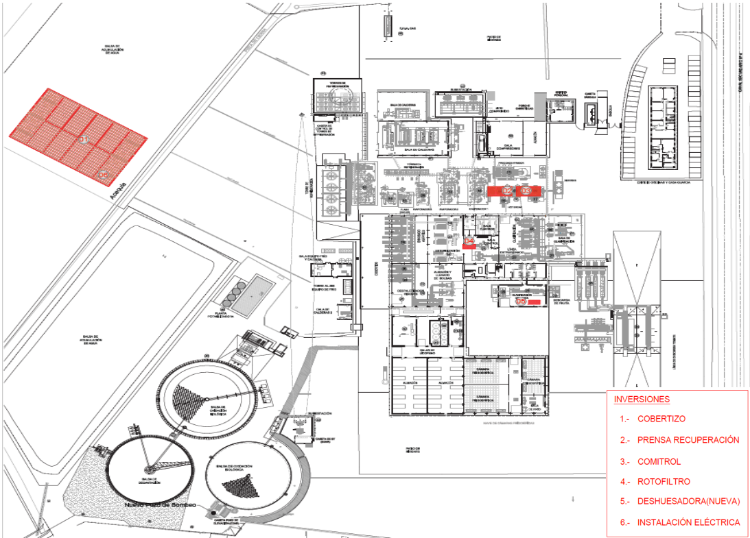
Plano I. Estado proyectado tras la modificación. (Fuente: Documento ambiental)
